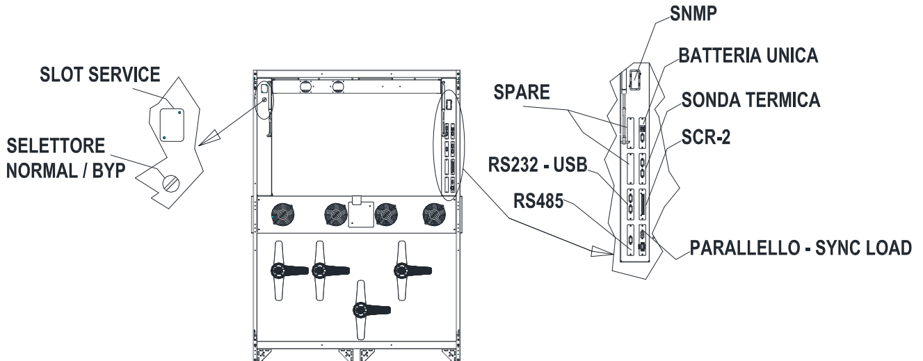
Figura 8 – Posizione schede di interfaccia INGENIO MAX 400-500 kVA
