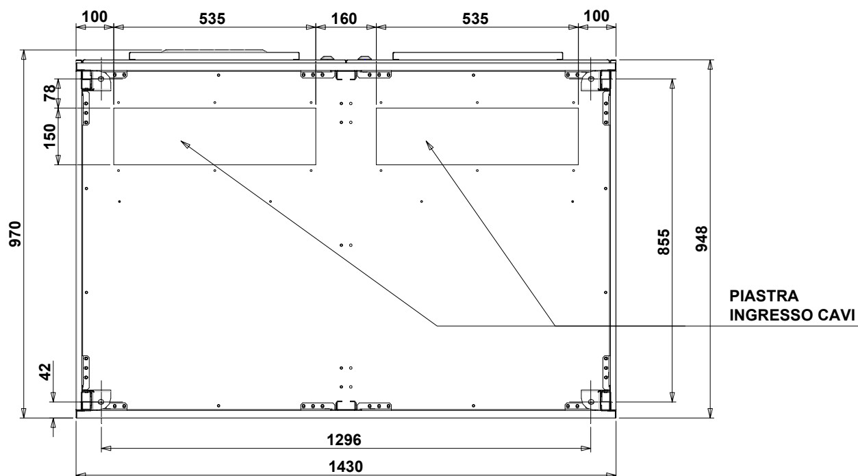
Figura 3 – Pianta di base
