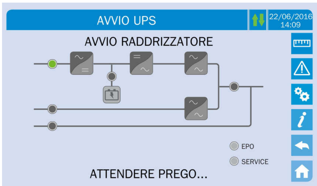
Figura 11 – Avvio raddrizzatore
