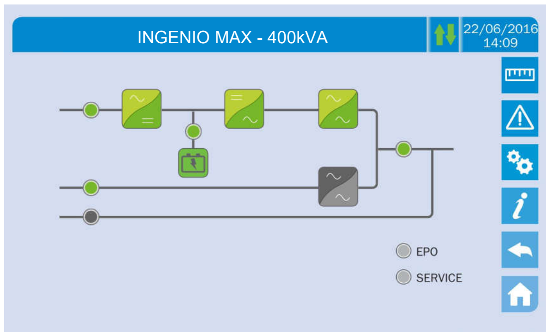
Figura 24 – Avvio da bypass manuale completato
