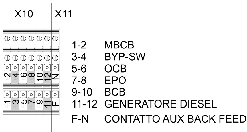
Figura 7 – Morsetti ausiliari INGENIO MAX 400-500 kVA
