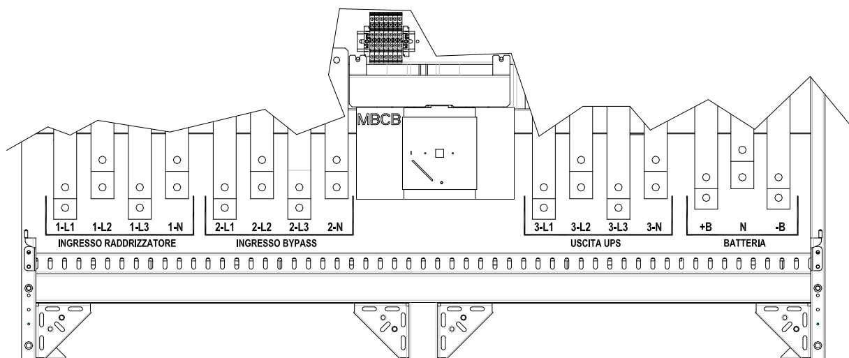
Figura 6 – Morsettiera INGENIO MAX 400-500 kVA
