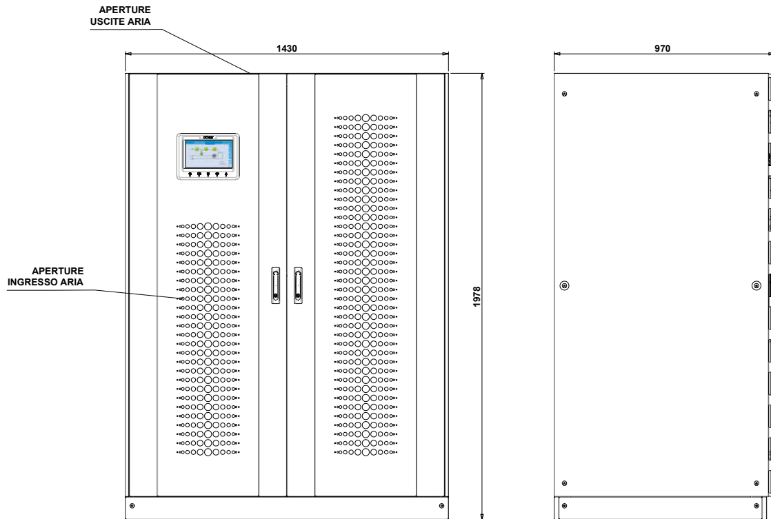
Figura 4 – Dimensioni di ingombro
