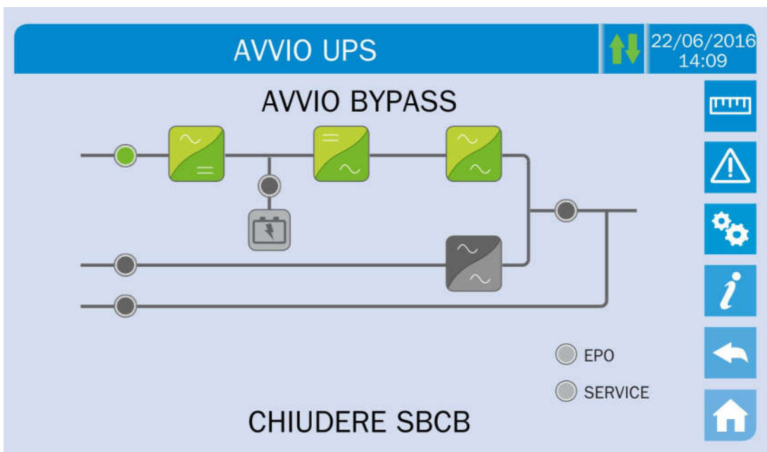
Figura 13 – Avvio bypass
