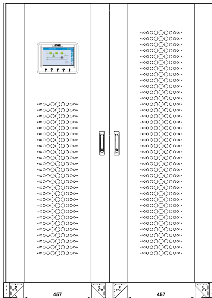
Figura 2 – Movimentazione UPS INGENIO MAX 400-500 kVA
