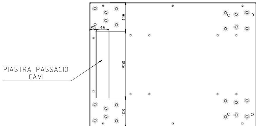
Figura 3 – Pianta di base
