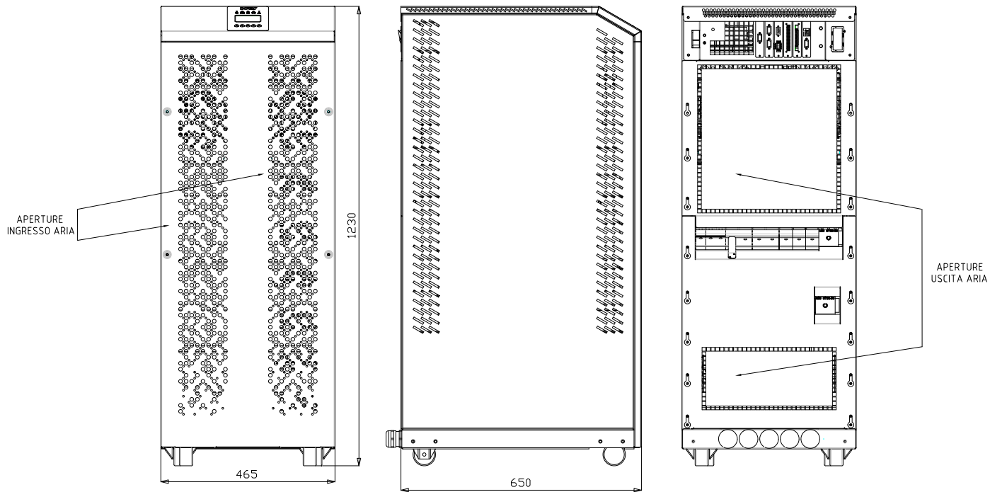
Figura 4 – Dimensioni di ingombro
