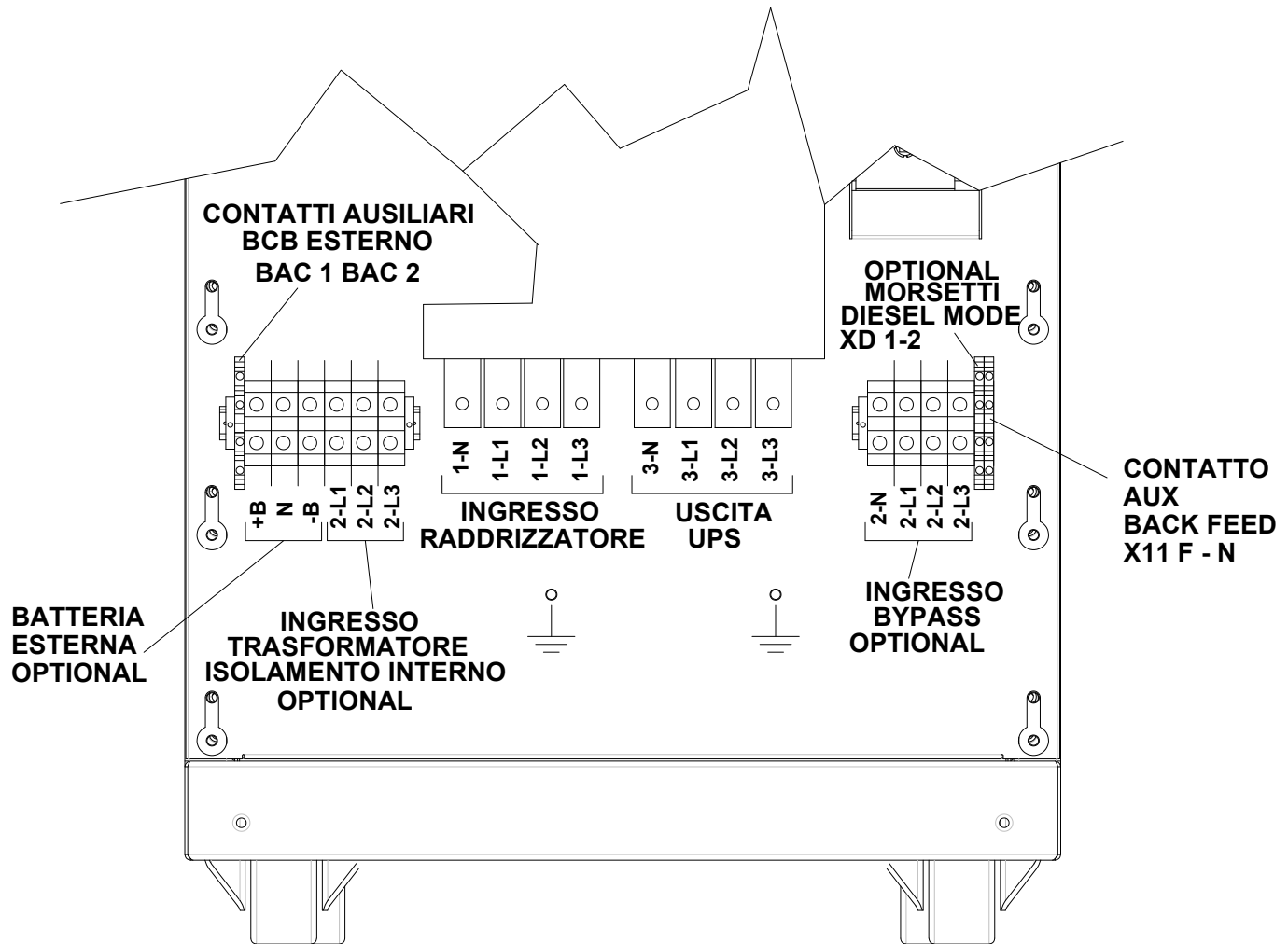
Figura 7 – Morsettiera INGENIO PLUS 40 kVA
