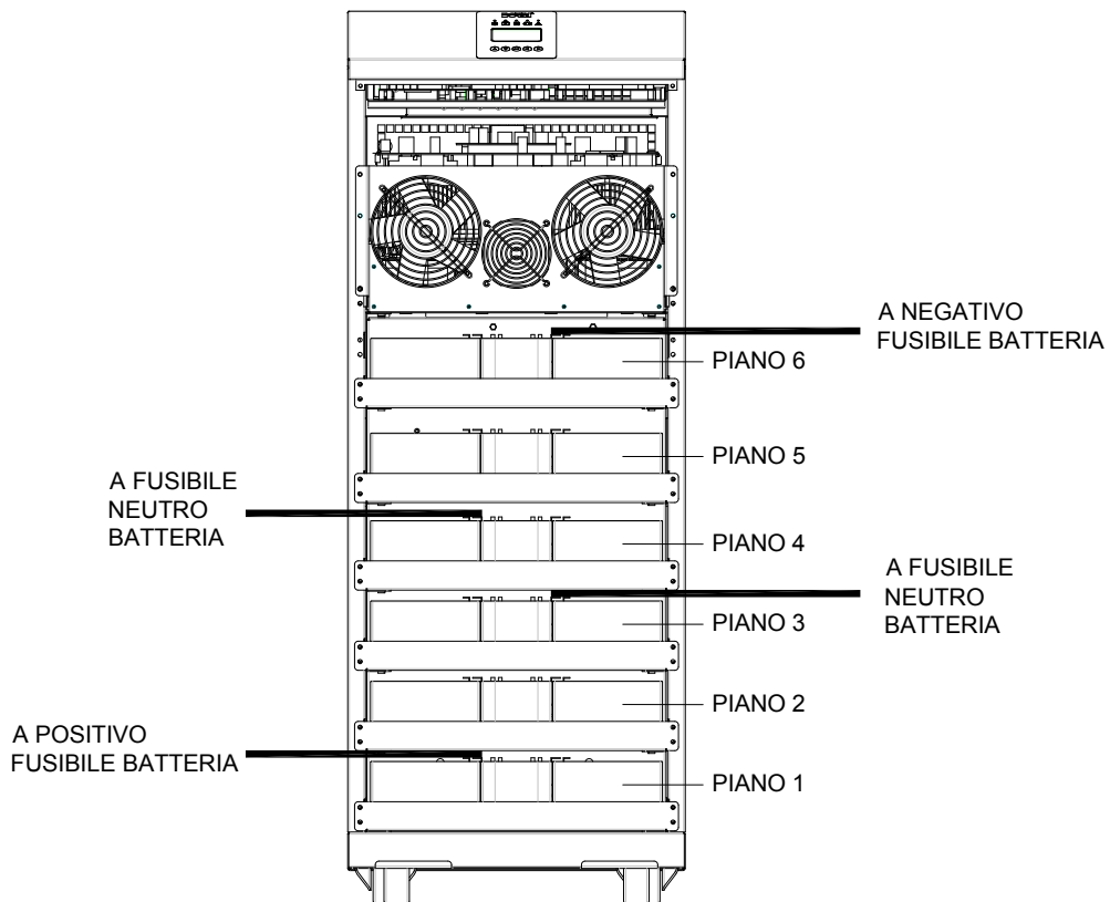
Figura 16 - 60 x 12Ah 12V connessione vassoi batterie vista frontale
