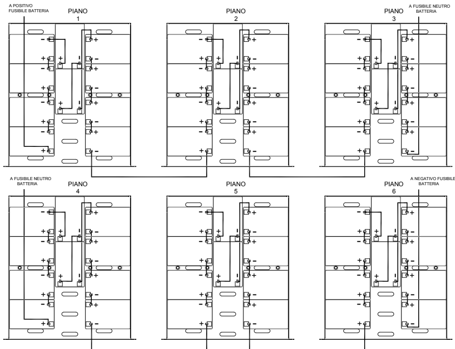
Figura 15 - 60 x 12Ah 12V connessione vassoi batterie vista dall'alto
