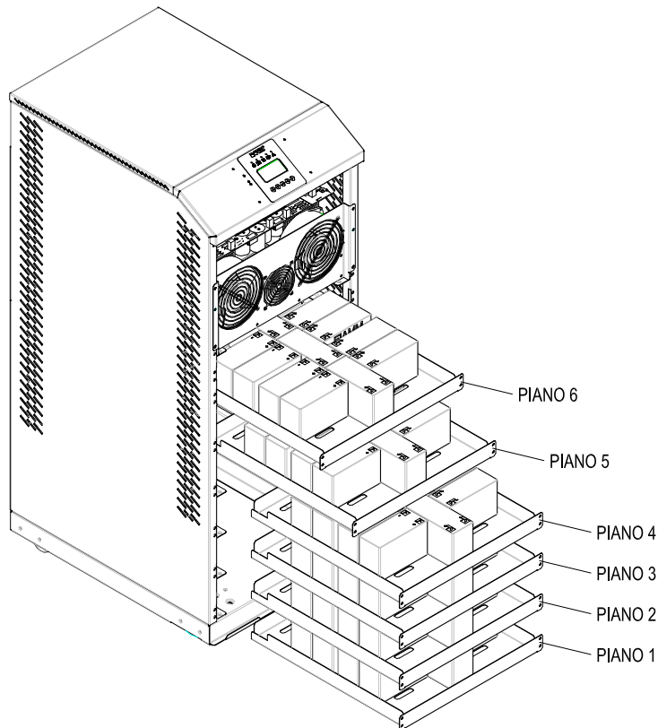
Figura 13 – Vassoi batterie 60 x 12Ah 12V vista laterale
