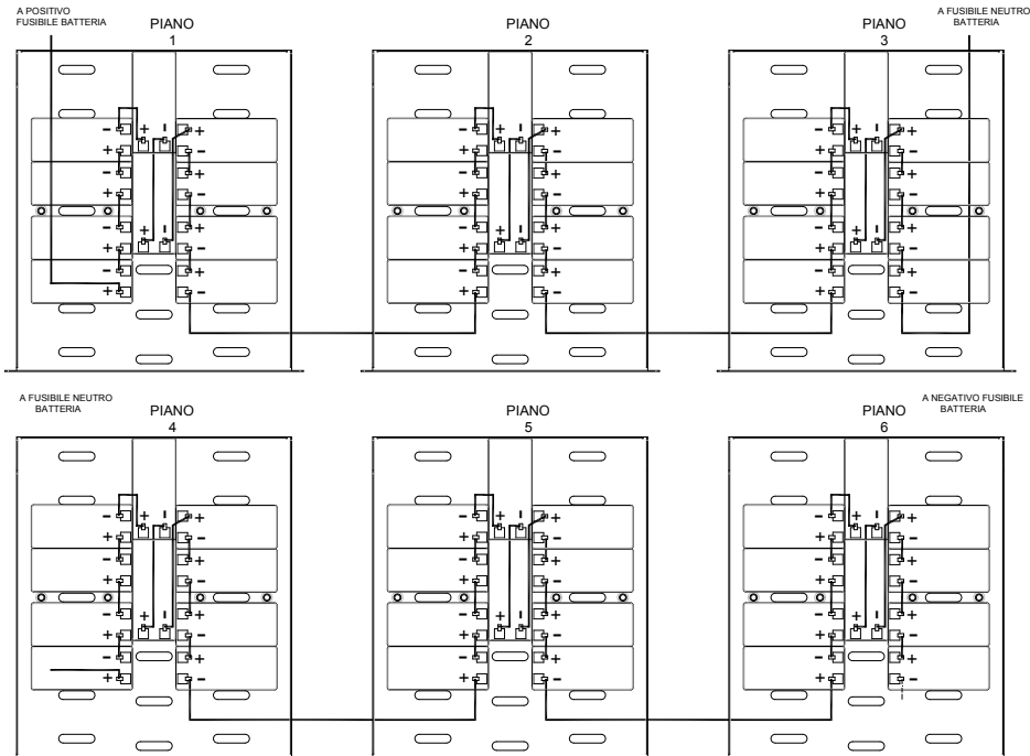
Figura 11- 60 x 9Ah 12V connessione vassoi batterie vista dall'alto
