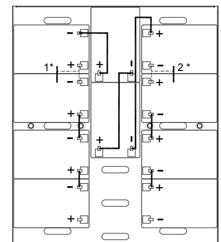
Figura 13 – Vassoi batterie 60 x 12Ah 12V vista laterale
