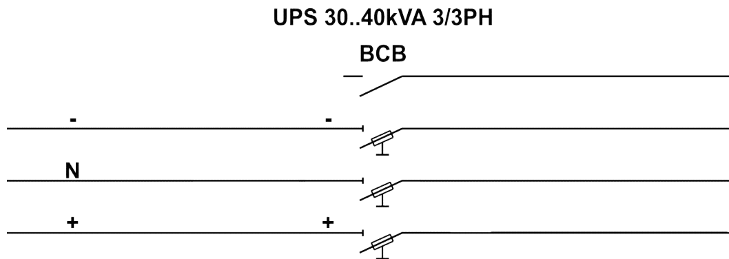
Figura 8 – Cablaggio portafusibili BCB
