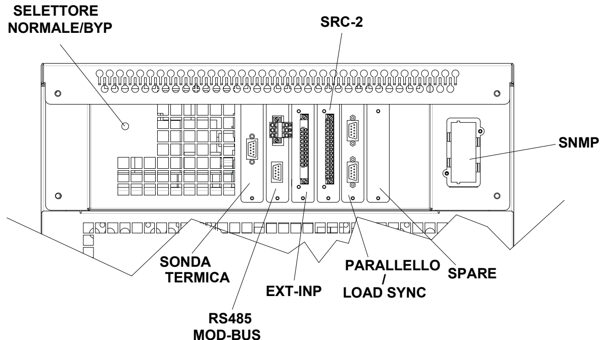
Figura 17 – Posizione schede di interfaccia
