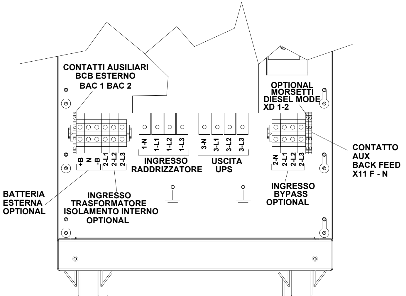
Figura 6 – Morsetti INGENIO PLUS 30 Kva
