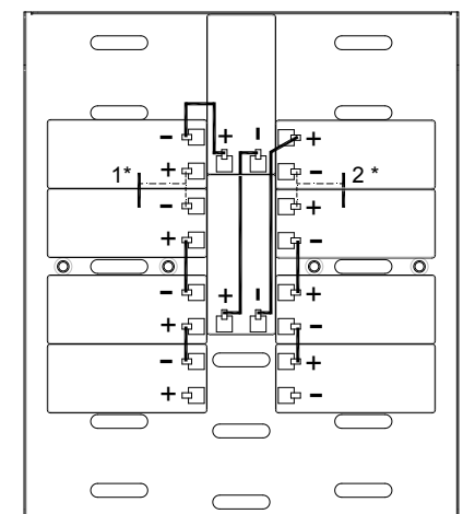
Figura 9 – Vassoi batterie 60 x 9Ah 12V vista laterale
