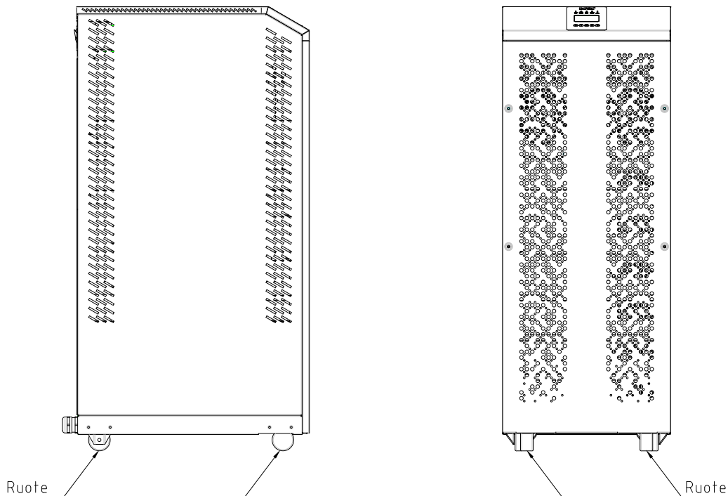
Figura 2 – Movimentazione UPS INGENIO PLUS 30÷40 kVA
