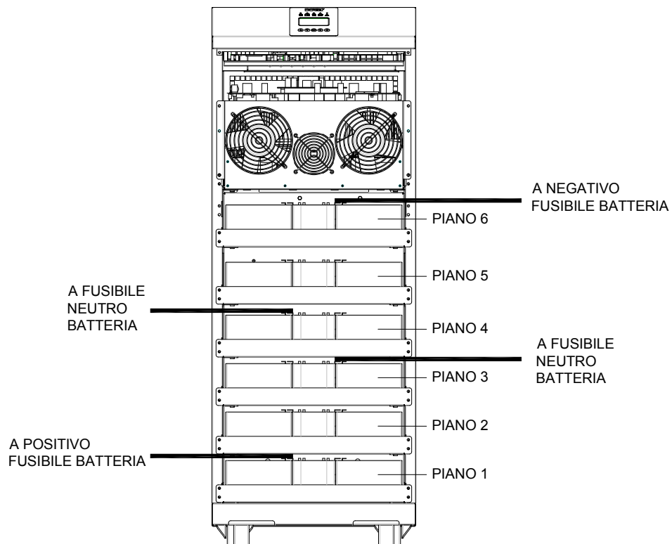
Figura 12- 60 x 9Ah 12V connessione vassoi batterie vista frontale
